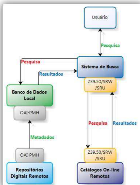
Figura 2 – Modelo de integração dos protocolos.
