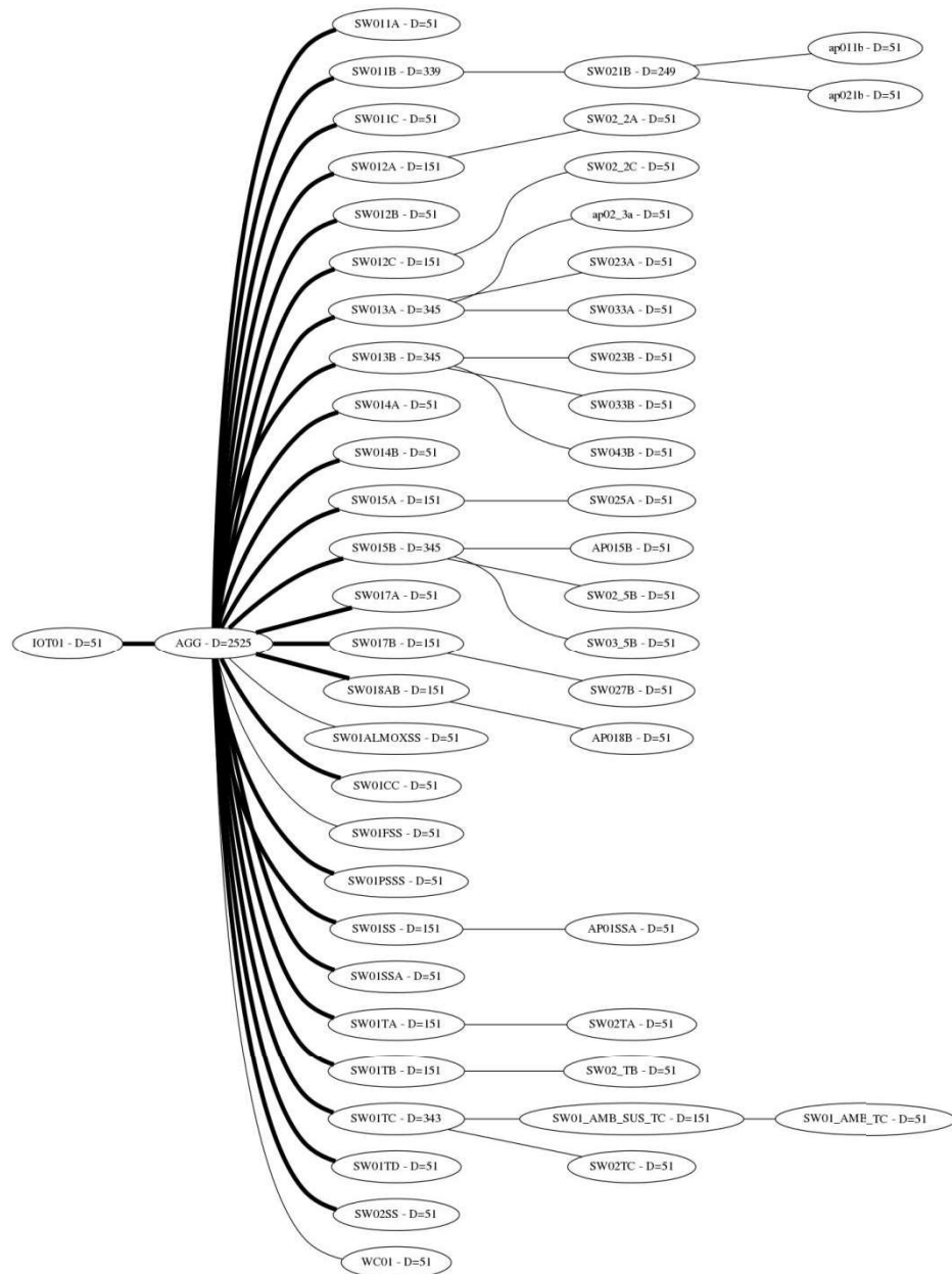
Figura 49: Diagrama da rede onde se encontra em cada balão o nome do nó e o seu respectivo grau de centralidade D .
