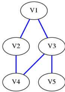
Figura 48: representação de um grafo G , cuja ordem e tamanho são 5.
